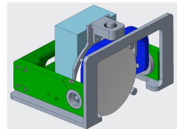
Abbildung 1: Präzisionsspiegelaufhängung
